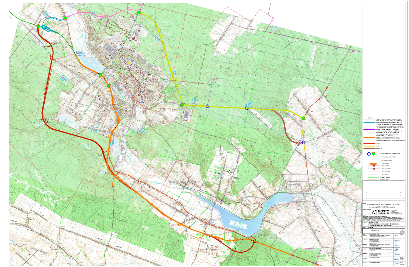
Warianty przebiegu obwodnicy Starachowic - orientacja
